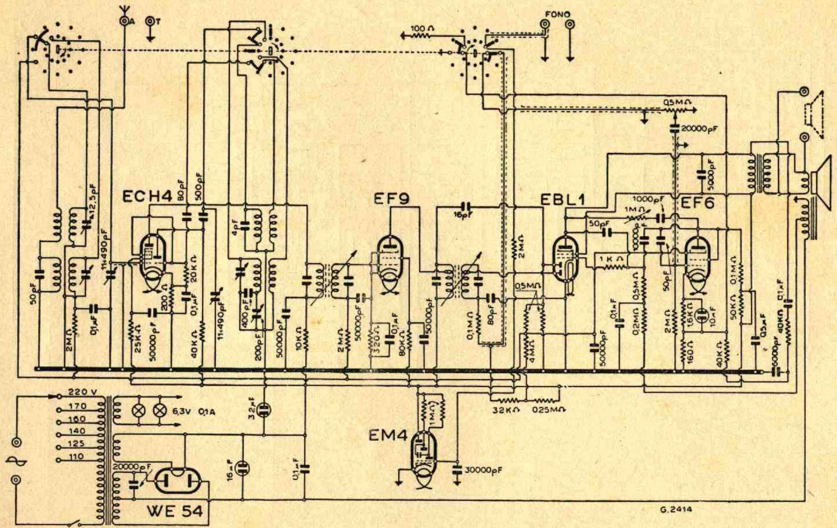
Lo schema elettrico del mod. 466
